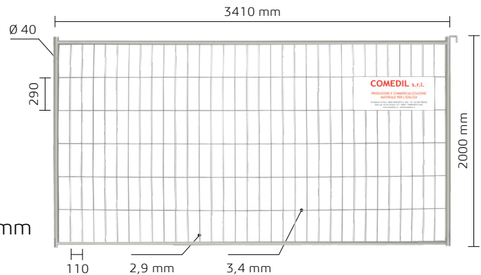
Pannello con 4 pali a rete liscia
